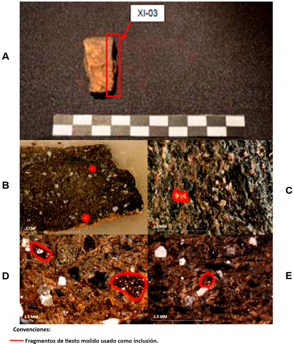
Figura 5. Petrografía de fragmento del grupo 3: (A) foto del fragmento que indica área de corte; (B) detalle de testigo; (C) vista de matriz con baja recristalización; (D) detalle de granulometría de los desgrasantes, y (E) detalle de la presencia de grietas internas en la matriz arcillosa
