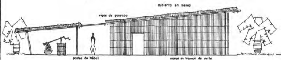
ALZADA B-B
